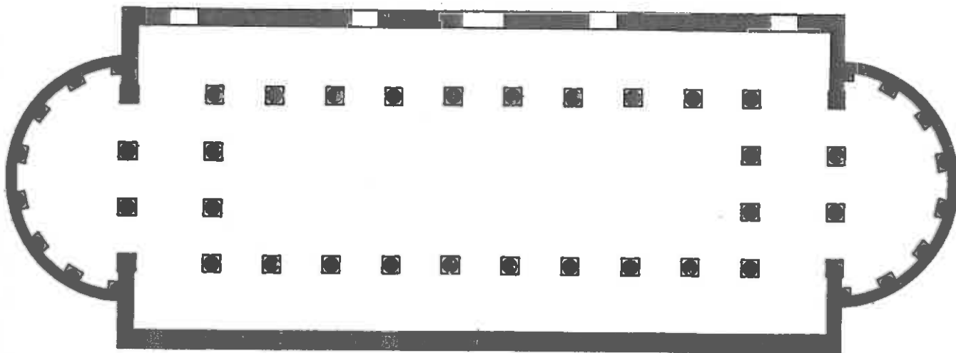
ichnographia basilicae Augustae Rauracorum prope Basileam sitae
