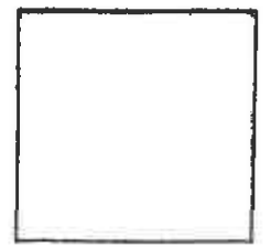
quadratum
