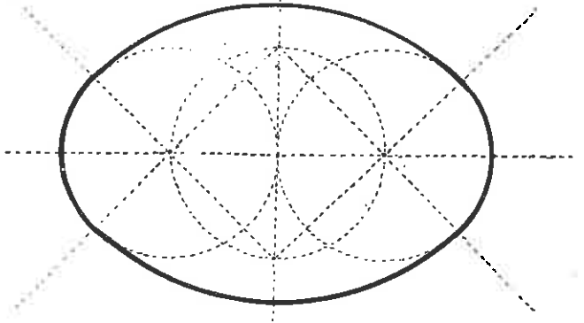
ovalis
