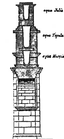
sectio Portae Sti. Laurentii, per cuius superiorem partem tres aquae ducuntur: aqua Iulia, aqua Tepula, aqua Marcia
