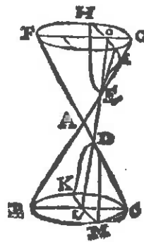
Hyperbola.
