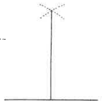
perpendicularis
